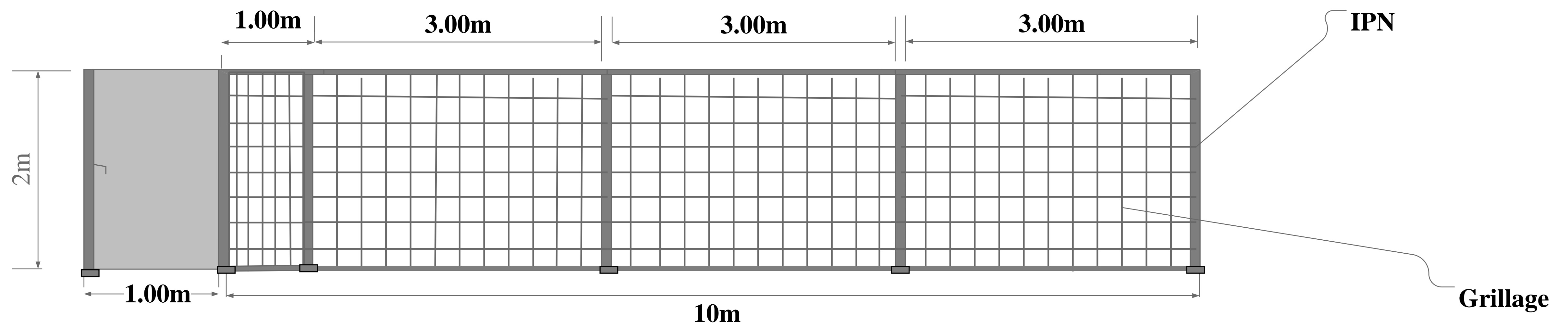
Vue principale(Vue de face) de la Clôture
