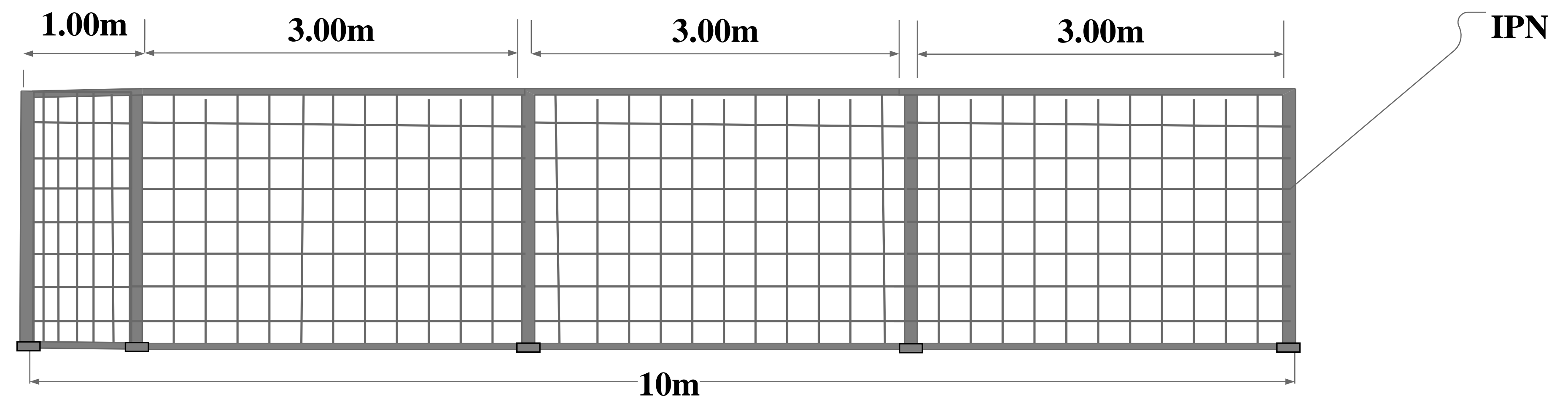
Vue de coté (gauche) de la clôture grillagée
